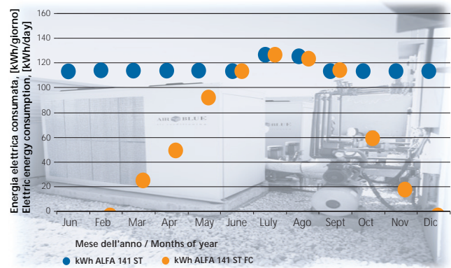
Località / Town Munich , potenza richiesta / power required 30 kW , temperatura acqua ingresso input water temperature 15°C , percentuale di glicole / glycol percentage 30% , funzionamento giorni settimana / operation days per week 7 , funzionamento ore giorno / operation hours a day 24 , consumo tot ALFA ST / tot. consump. ALFA ST 44006 kWh , consumo tot ALFA ST FC / tot. consump. ALFA ST FC 22797 kWh , risparmio percentuale / savings (percentage) 48% ,
