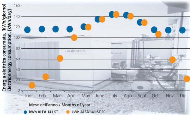
Località / Town Padova , potenza richiesta / power required 30 kW , temperatura acqua ingresso input water temperature 15°C , percentuale di glicole / glycol percentage 30% , funzionamento giorni settimana/operation days per week 7 , funzionamento ore giorno / operation hours a day 24 , consumo tot ALFA ST / tot. consump. ALFA ST 46597 kWh , consumo tot ALFA ST FC / tot. consump. ALFA ST FC 34040 kWh , risparmio percentuale / savings (percentage) 27% ,
